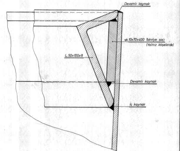
A - TAFSİLATI
